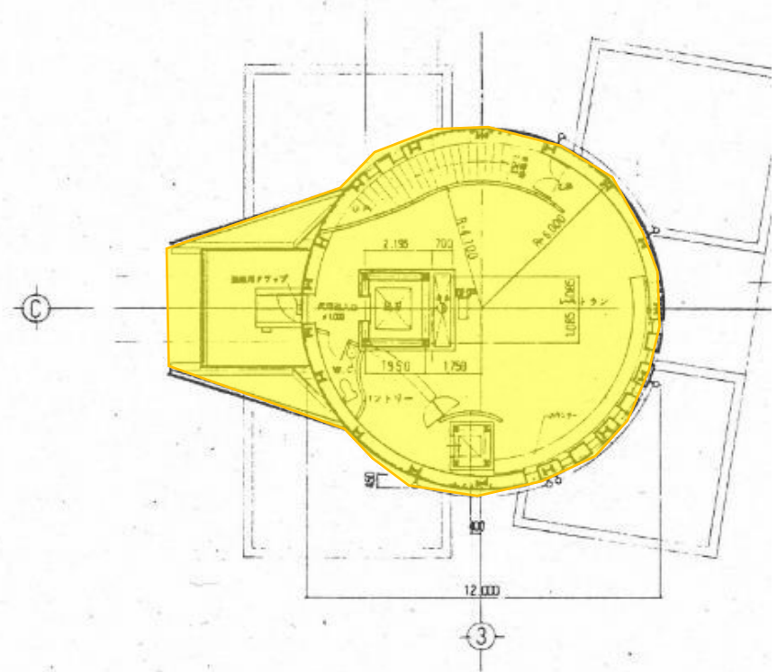
4階 平面図
