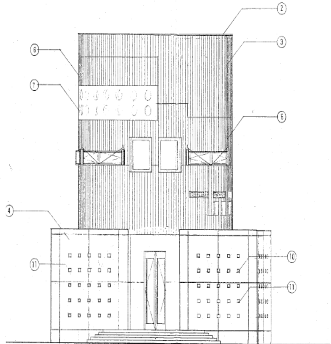
南側 立面図
