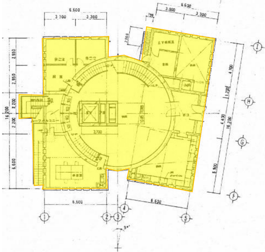
M2階平面図
