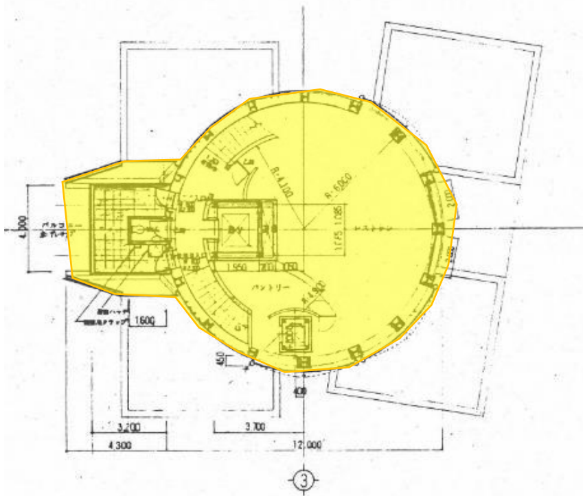
3階 平面図
