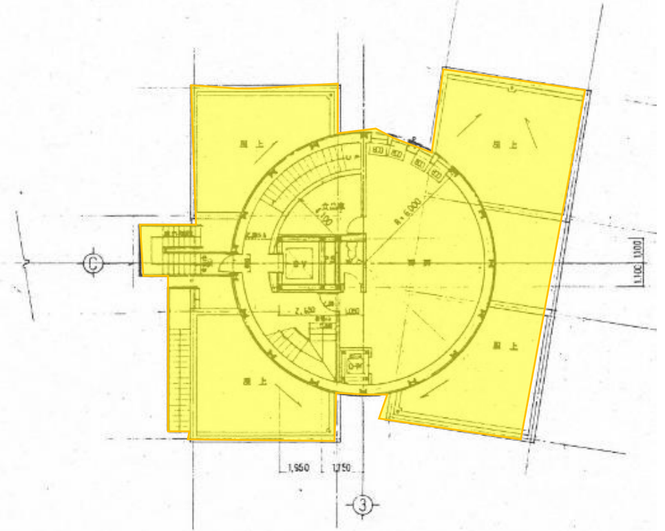
2階 平面図
