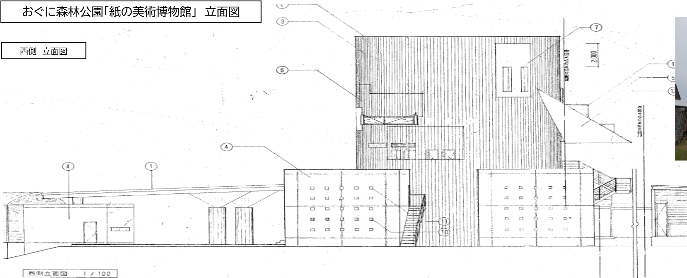
西側立面図 1 / 100
