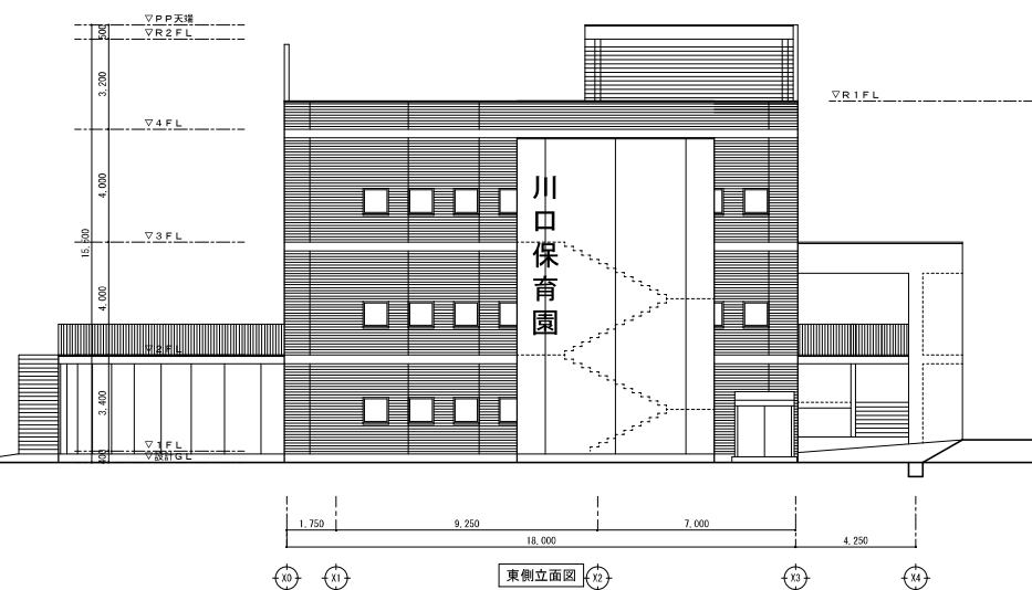
東側立面図
