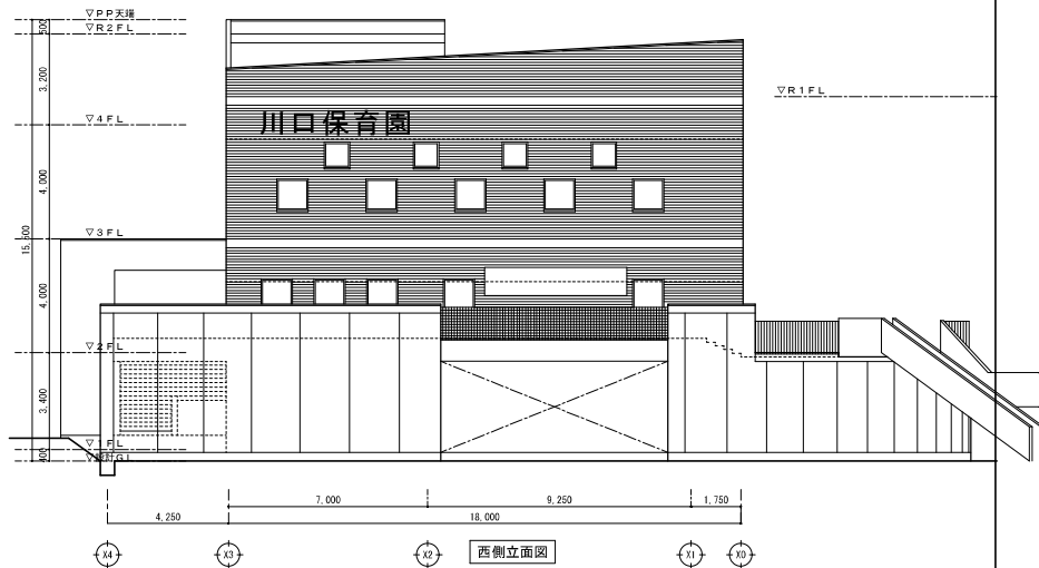
西側立面図
