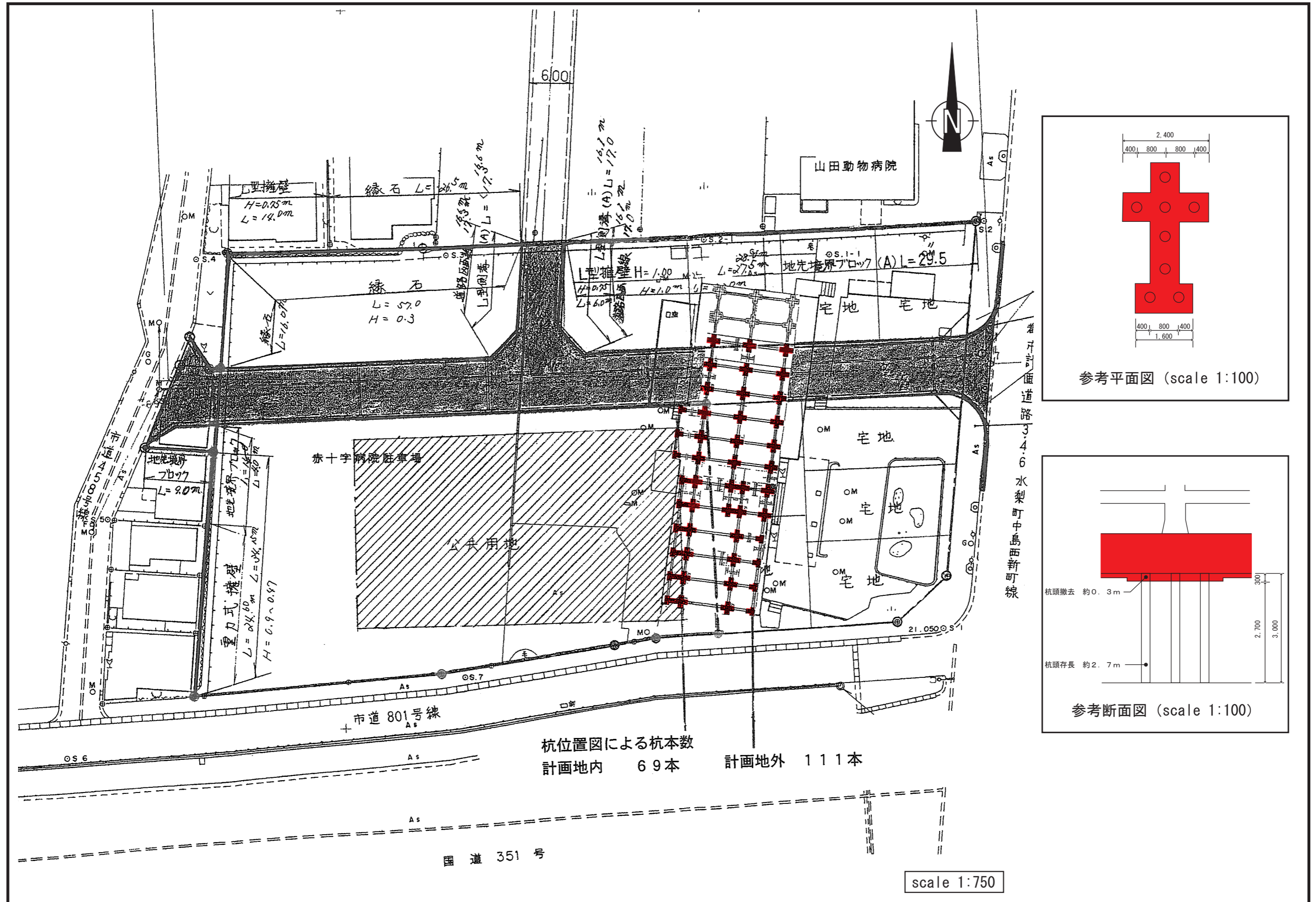
才. 旧建築物の埋設杭位置図
