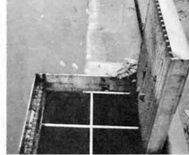
安全性を考えた投雪口(川崎6)
