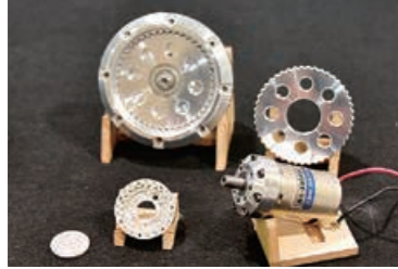
前列が同社製作の減速機の部品とそれを搭載したモーター（左下は1円玉）。後列が従来品
