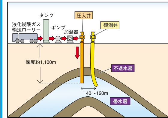
◀地下貯留の模式図
