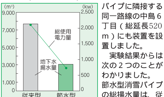
従来型と節水型の消雪ポンプの比較（同一面積の道路の消雪に要した地下水揚水量と電力量）
