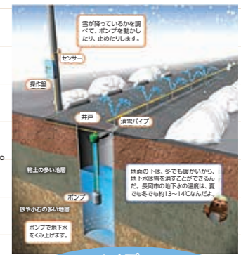
消雪パイプのしくみ
