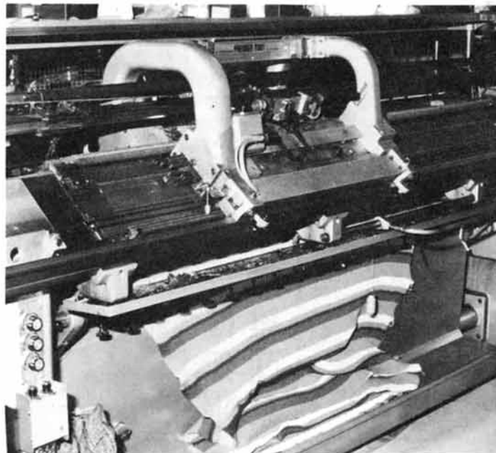
丸編のニットジャージ コンピューター化された横編機
