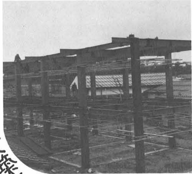
鉄骨が組立てられる (6月25日撮影)
