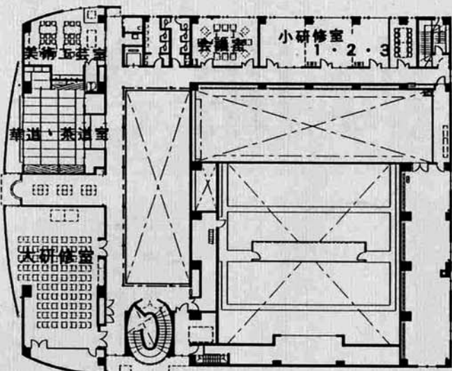
3階平面図
