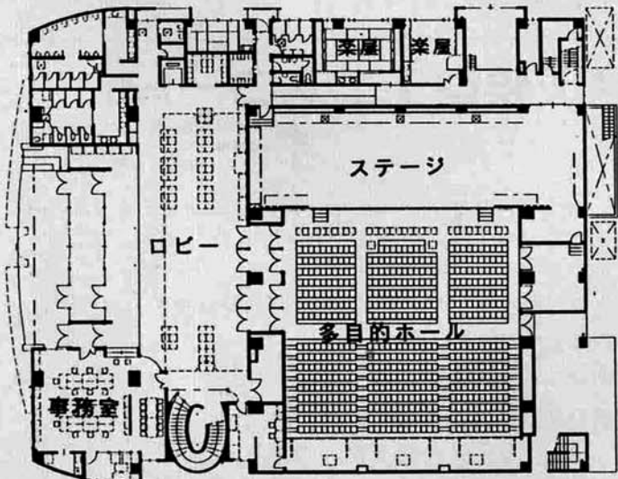
1階平面図
