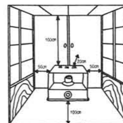
石油ストーブ(放射形)
