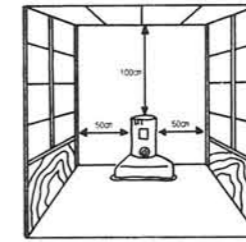
石油ストーブ(対流形)
