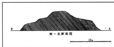
図52 鳥越経塚測量図(昭53.8.21)三島町史より
