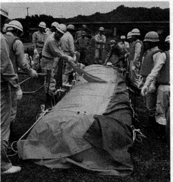
▲木流し工(越路町消防団) 洪水により堤防が洗掘されたり、洗掘されそうな場合に流水の勢いを減じ、法崩れを防ぐ工法
