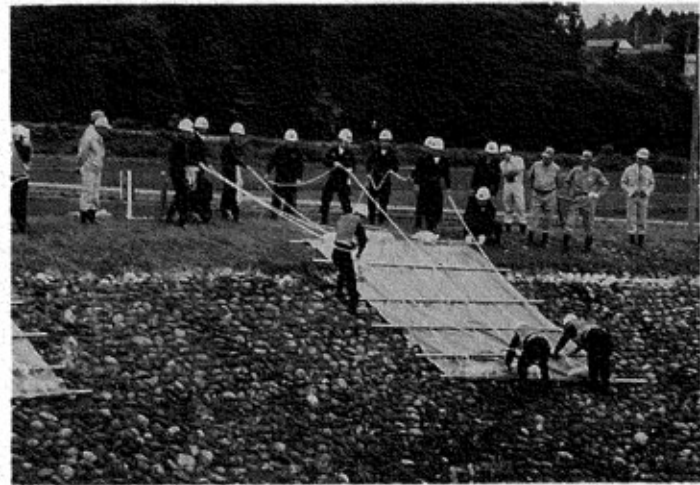
▲シート張り工(小千谷市消防団) 堤防法面の崩壊及び堤防の浸透水を防ぐため、ビニールシートで流水を遮断する工法
