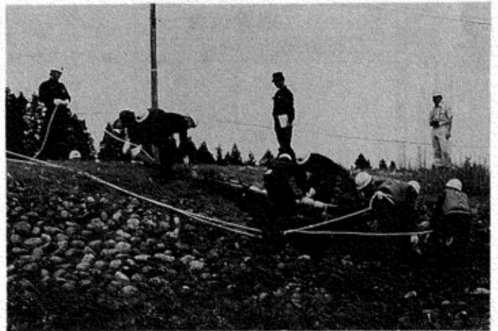
▲木流し工(越路町消防団) 洪水により堤防が洗掘されたり、洗掘されそうな場合に流水の勢いを減じ、法崩れを防ぐ工法
