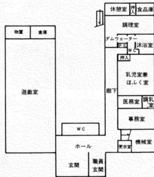
一階平面図
